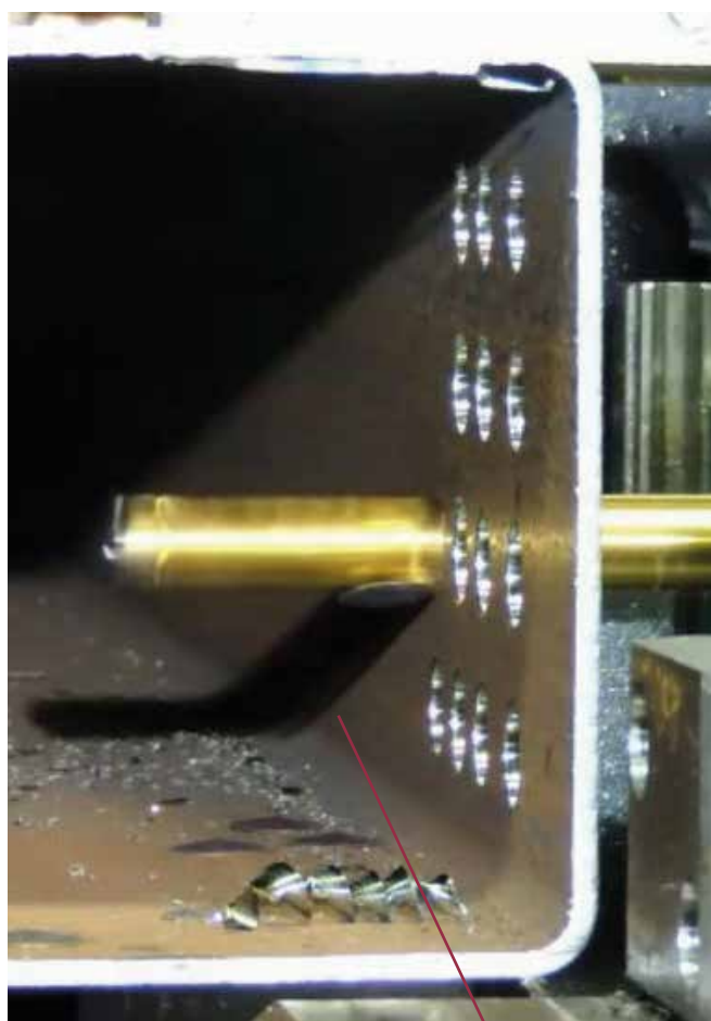
Capsule de perçage Drilling slug
